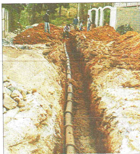
Instalação de manilhas no Bairro Retto Júnior
